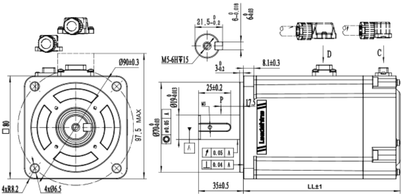
Dimensions
