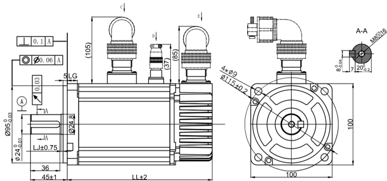
Dimensions
