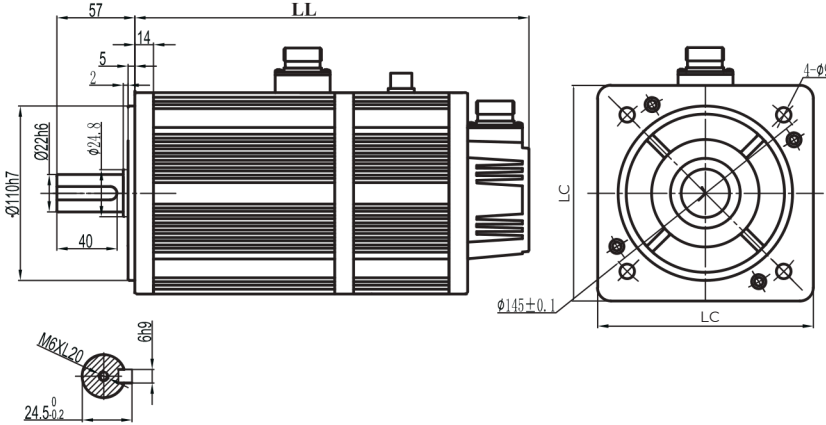
Dimensions
