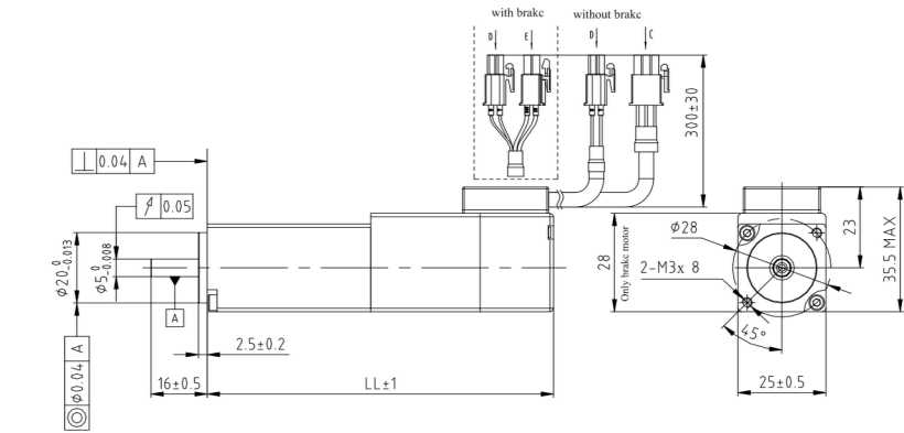
Dimensions
